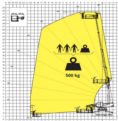
ROTEREND UITKLAPBAAR WERKPLATFORM 500 kg
